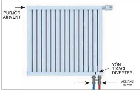
5- KOMPAKT ENTEGRE TERMOSTATİK VANALI BAĞLANTI
