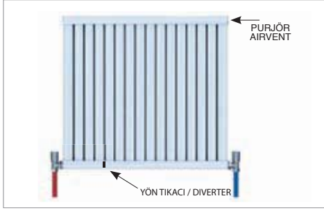
1- ALT KARŞIT UÇ BAĞLANTI
