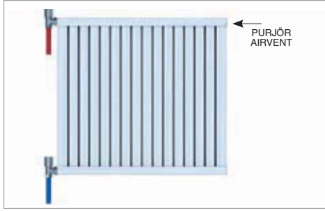
3- PARALEL BAĞLANTI
